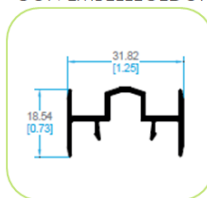
74639 UNIÓN CUATRO HOJAS CON EMBELLECEDOR
