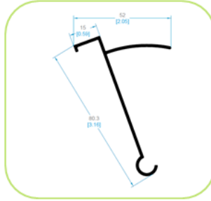
3518 ESQUINERO REGULABLE HEMBRA
