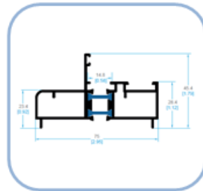
4653 FIJO DOS RIELES
