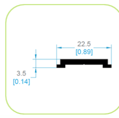
1506 PLETINA CREMONA
