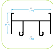
3502 CERCO SUPERIOR
