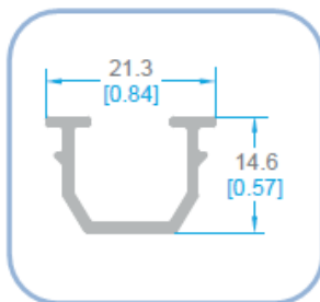
4605-P ADAPTADOR 10mm PVC
