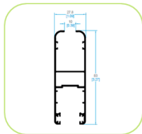
64622 HOJA PERIMETRAL MONUMENTAL
