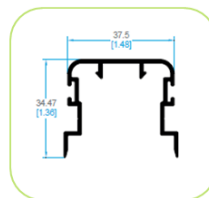
64614 TAPA DOBLE HOJA CENTRAL
