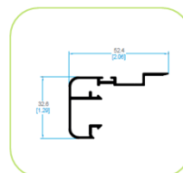
64630 TAPA HOJA CENTRAL MONUMENTAL CORTA
