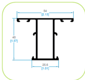
1400 PILASTRA LISA VENTANA/ HOJA APERTURA EXTERIOR
