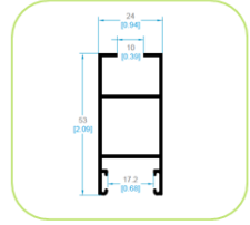
3505 HOJA LATERAL
