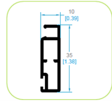
3535 HOJA LATERAL MOSQUITERO
