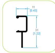
3534 GUÍA MOSQUITERO
