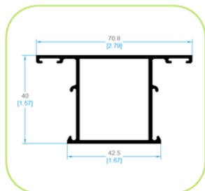
1405 PILASTRA LISA PUERTA/ HOJA APERTURA EXTERIOR
