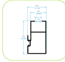
3504 HOJA CENTRAL
