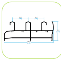
4602 MARCO PERIMETRAL 3 RIELES
