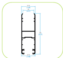
64621 HOJA PERIMETRAL DOBLE VIDRIO
