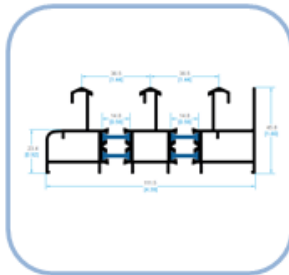
4652 MARCO TRES RIELES
