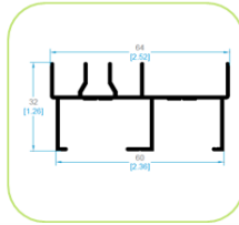
3508 CERCO LATERAL
