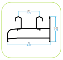
74631 MARCO PERIMETRAL RECTO
