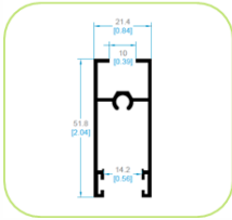
3507 HOJA DE RUEDAS
