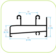
3501 CERCO INFERIOR
