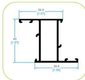
1401 HOJA LISA VENTANA/ APERTURA INTERIOR
