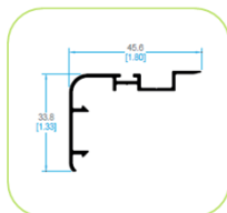
64620 TAPA HOJA CENTRAL MONUMENTAL
