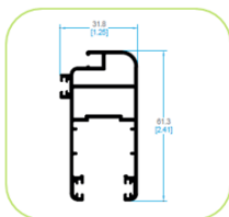
64624 HOJA PERIMETRAL MOSQUITERO
