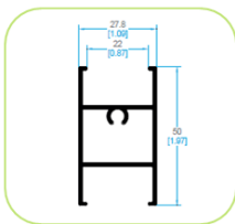
4608 INTERMEDIO DOBLE VIDRIO
