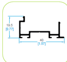
61446 ARRASTRE PUERTA
