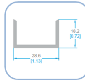
4651-P CANAL MARCO PVC
