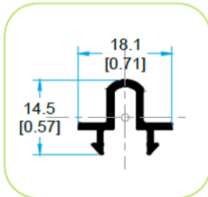
3609 UNIÓN 4 HOJAS
