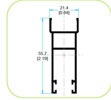
3606 HOJA PERIMETRAL DOBLE VIDRIO
