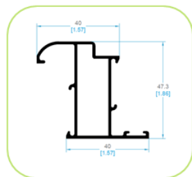
1403 HOJA CURVA VENTANA/ APERTURA INTERIOR
