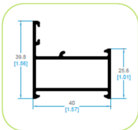
1402 MARCO LISO VENTANA
