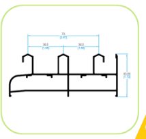
74632 MARCO PERIMETRAL TRES RIELES RECTO
