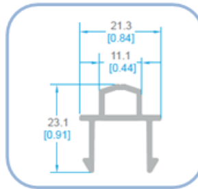
4609-P UNIÓN CUATRO HOJAS PVC
