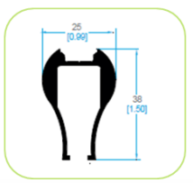
4611 TIRADOR REFUERZO
