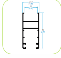
4606 HOJA PERIMETRAL DOBLE VIDRIO
