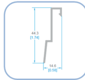
4654-P UNIÓN HOJA CENTRAL PVC
