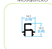
4610 ADAPTADOR MOSQUITERO
