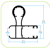
4627 HOJA PERIMETRAL PLAYA REFORZADA
