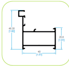
61449 MARCO CON MOSQUITERO
