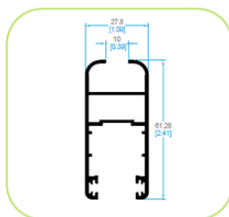
64628 HOJA PERIMETRAL LISA
