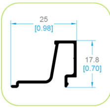
61448 JUNQUILLO 24mm
