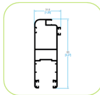
64623 HOJA PERIMETRAL MOSQUITERO MONUMENTAL
