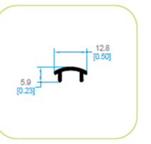
4612 TAPA TIRADOR REFUERZO
