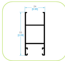
3555 HOJA LATERAL DOBLE VIDRIO
