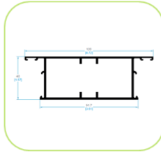
1423 HOJA MONUMENTAL EXTERIOR/ PILASTRA MONUMENTAL
