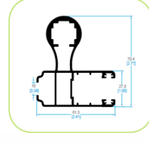
4625 HOJA PERIMETRAL REFORZADA
