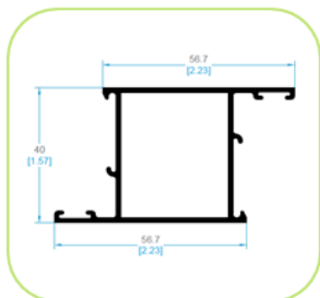
1406 HOJA LISA PUERTA/ APERTURA INTERIOR
