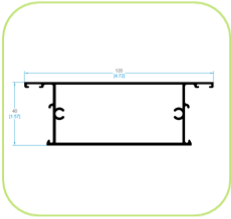
1422 ZÓCALO CENTRAL
