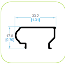
1428 ESQUINERO 45°
