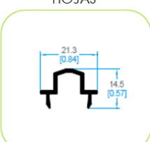
4609 UNIÓN CUATRO HOJAS
