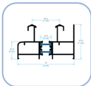
4651 MARCO DOS RIELES
