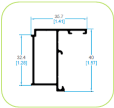
61447 INVERSOR DE APERTURA
