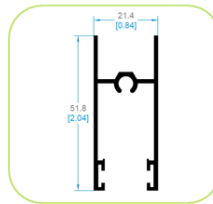
3557 HOJA DE RUEDAS DOBLE VIDRIO
