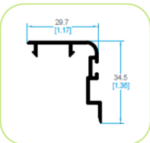
4604 TAPA HOJA CENTRAL
