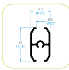
2416 CUADRÍCULA
