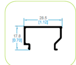
1430 JUNQUILLO ANCHO
