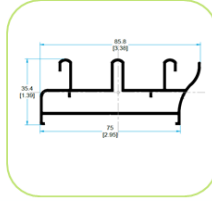
3604 TAPA HOJA CENTRAL
