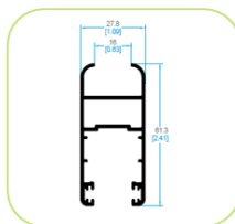
4615 HOJA PERIMETRAL PLAYA
