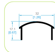
3513 TAPA CERCO LATERAL
