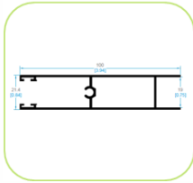
3560 ZÓCALO
