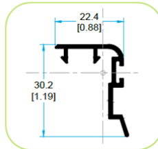
3604 TAPA HOJA CENTRAL
