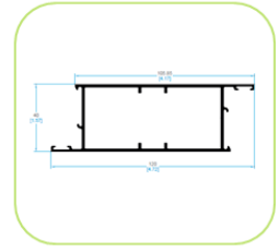
61445 HOJA MONUMENTAL INTERIOR
