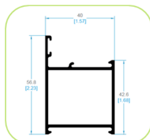
1407 MARCO LISO PUERTA
