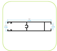
3559 ZÓCALO DOBLE VIDRIO
