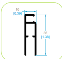
3536 HOJA RUEDA MOSQUITERO
