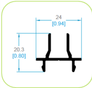
3517 UNIÓN DE CUATRO HOJAS
