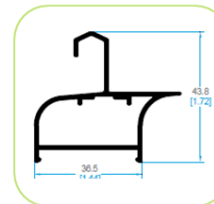
4633 MARCO ADAPTADOR
