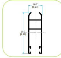
3605 HOJA PERIMETRAL
