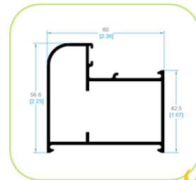
1408 MARCO CURVO PUERTA
