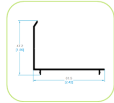
3512 SOLAPE EMBELLECEDOR
