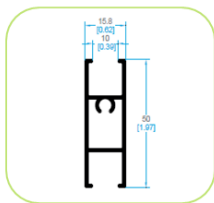
4607 INTERMEDIO
