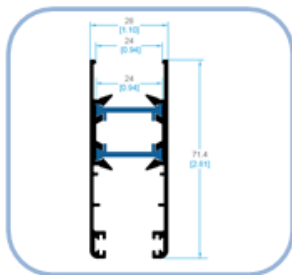
4656 HOJA PERIMETRAL
