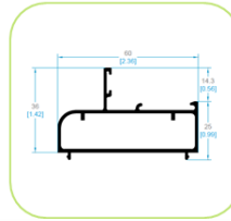
3510 FIJO TUBULAR
