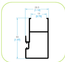
3554 HOJA CENTRAL DOBLE VIDRIO
