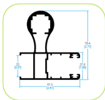
4626 HOJA PERIMETRAL DOBLE VIDRIO REFORZADA
