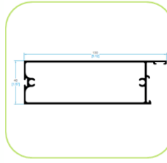
1434 ZÓCALO INFERIOR
