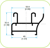
3609 UNIÓN 4 HOJAS
