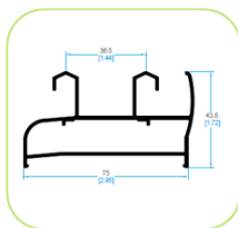
4601 MARCO PERIMETRAL
