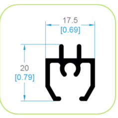
2415 RECERCADO
